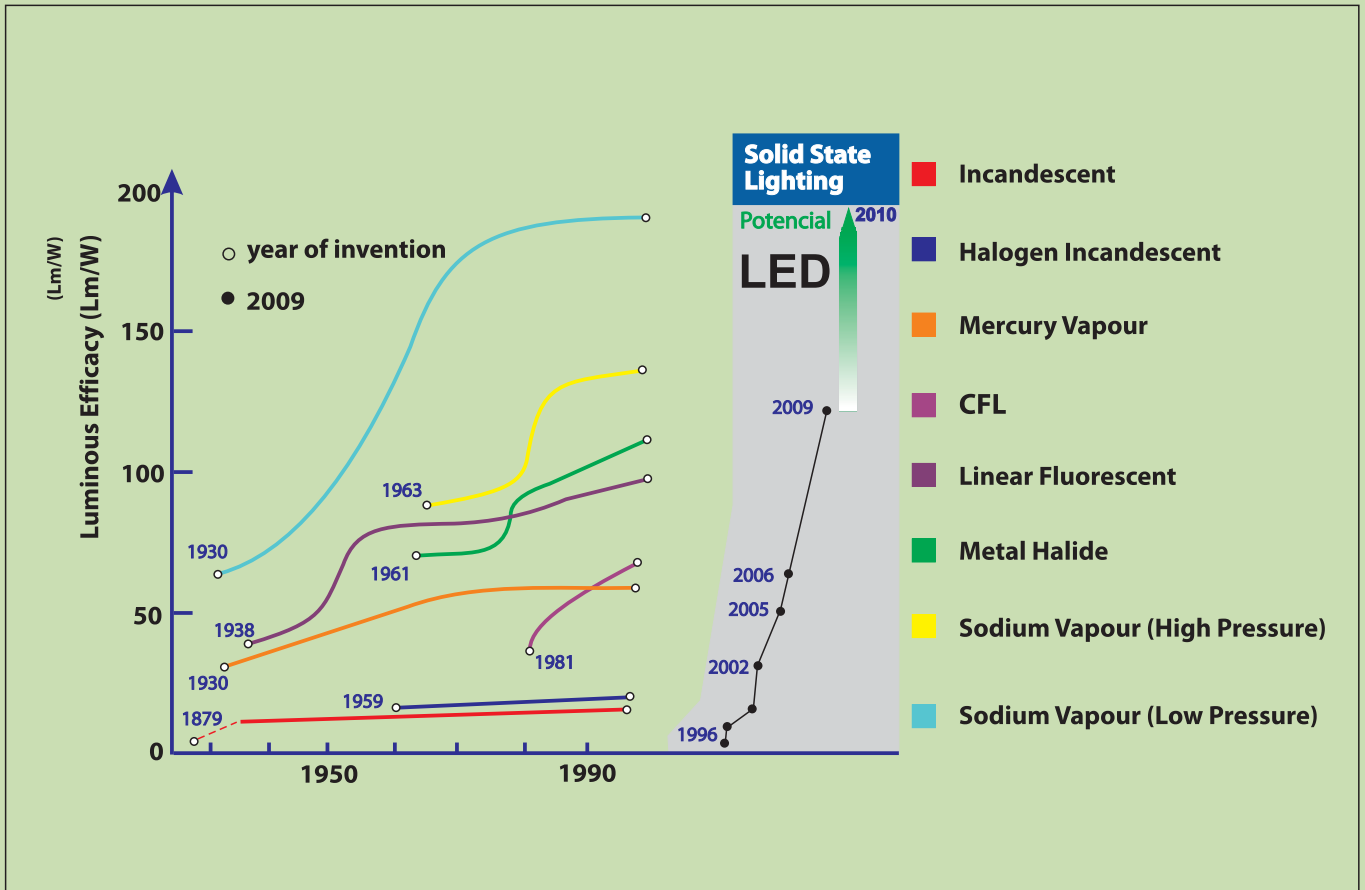
Rys. 1. Ewolucja wydajności świetlnej w różnych technologiach (źródło: de Almeida 2009 Technology Assessment, E4)
